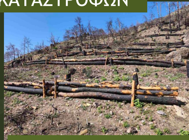
Έργα αντιδιαβρωτικής προστασίας στο Λασιθί
