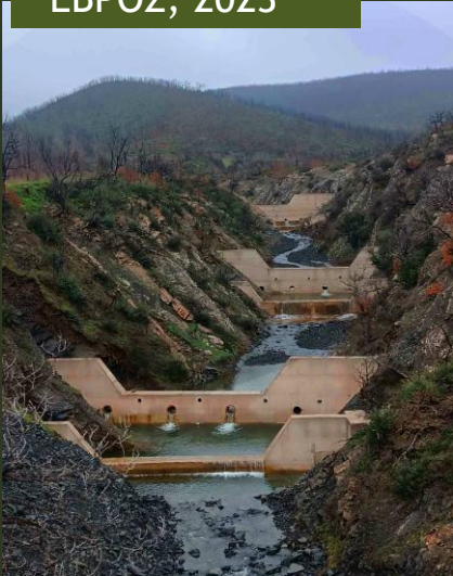
Ορεινά υδρονομικά έργα στον Έβρο
